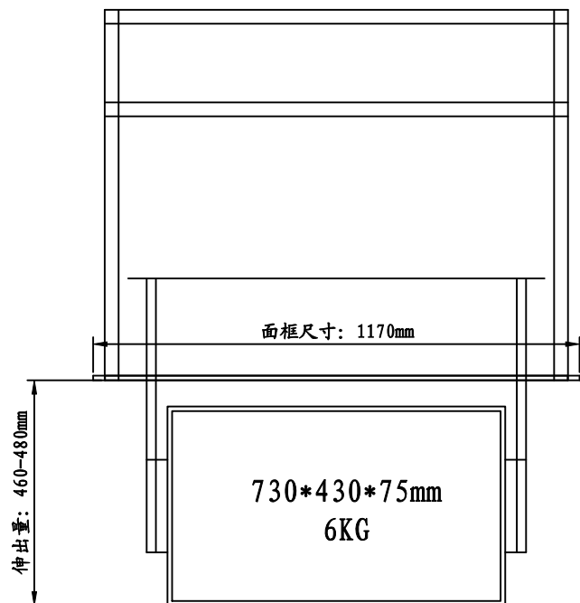
仰视图
