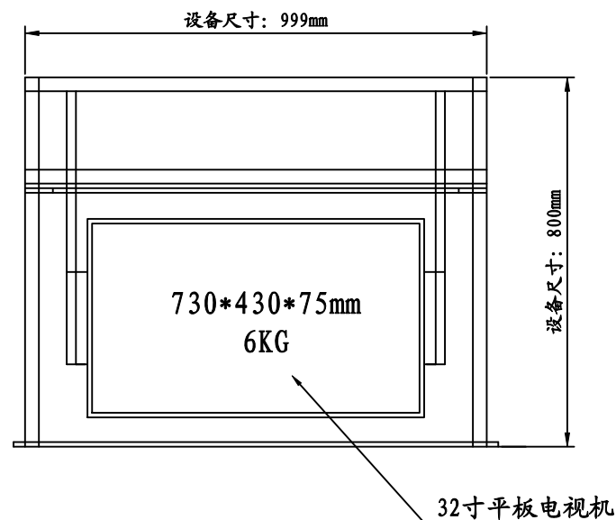
使用状态
