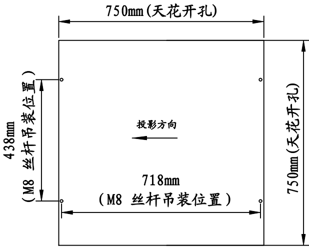
开孔及安装吊杆位置尺寸
