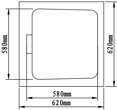
开孔及安装吊杆位置尺寸
