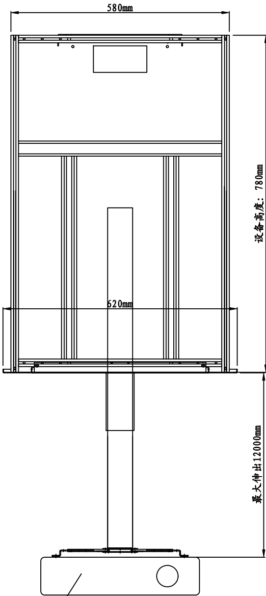
正视图 (投影机伸出时)
