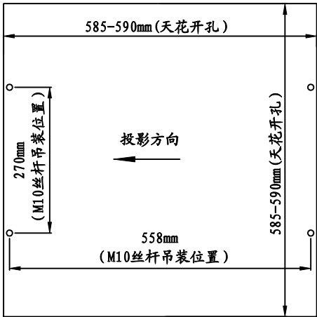
开孔及安装吊杆位置尺寸
