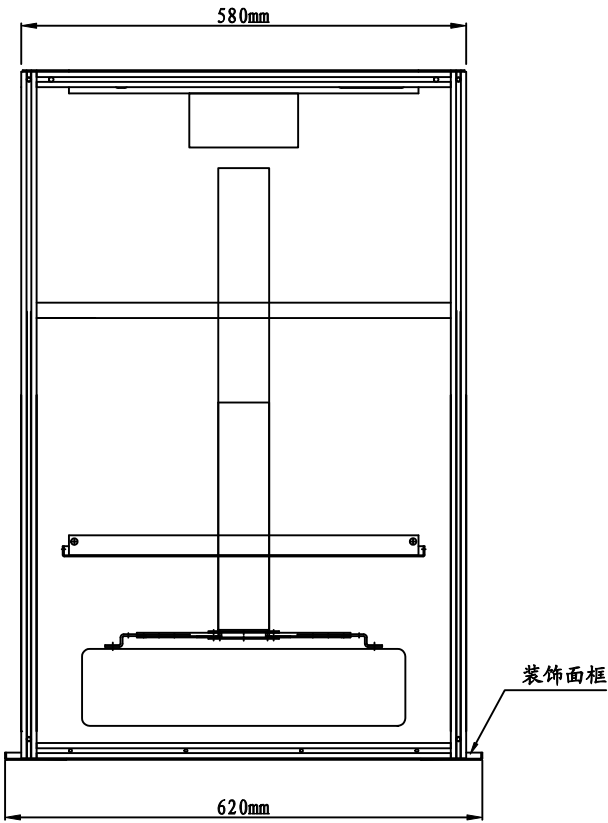
侧视图 (投影机隐藏时)
