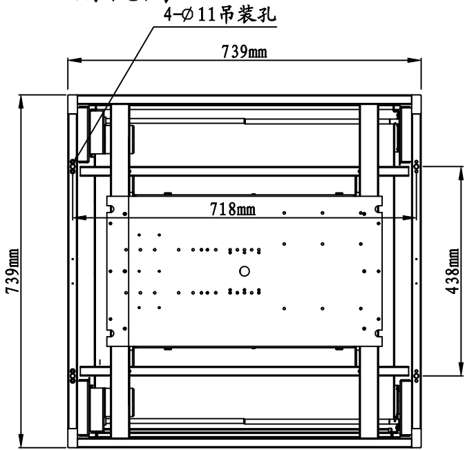
俯视图
